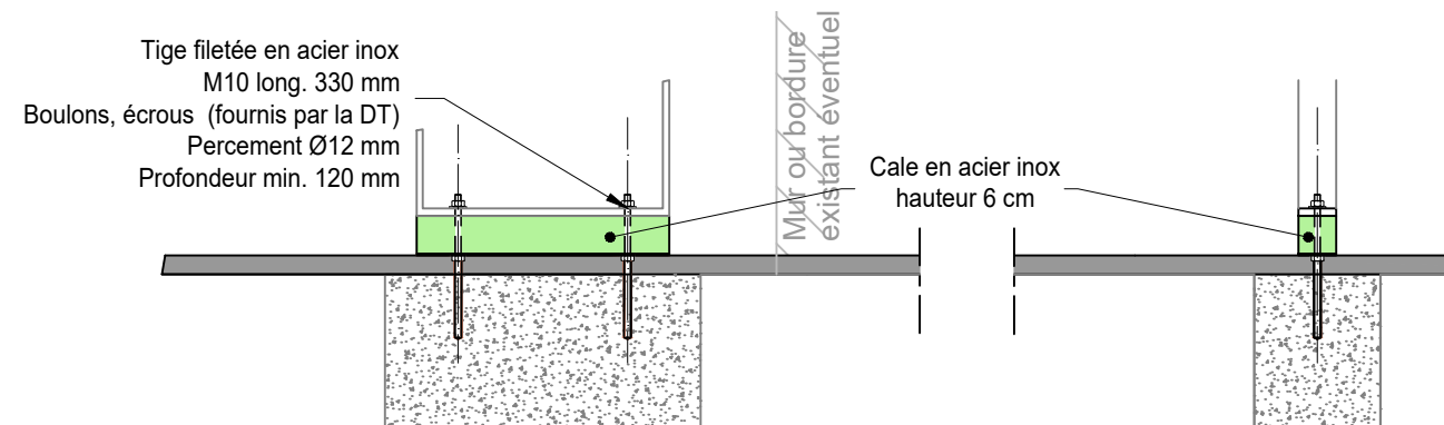
Détails de fixation
