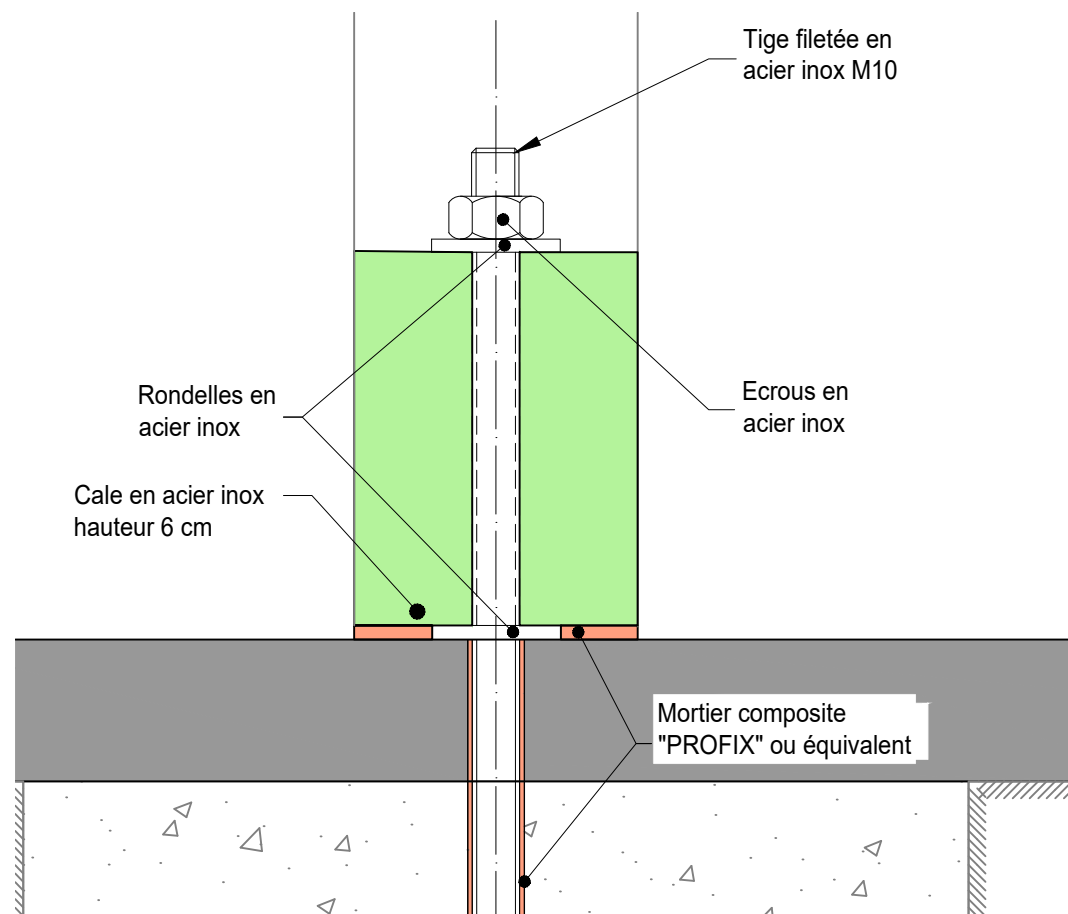
Détails de fixation
