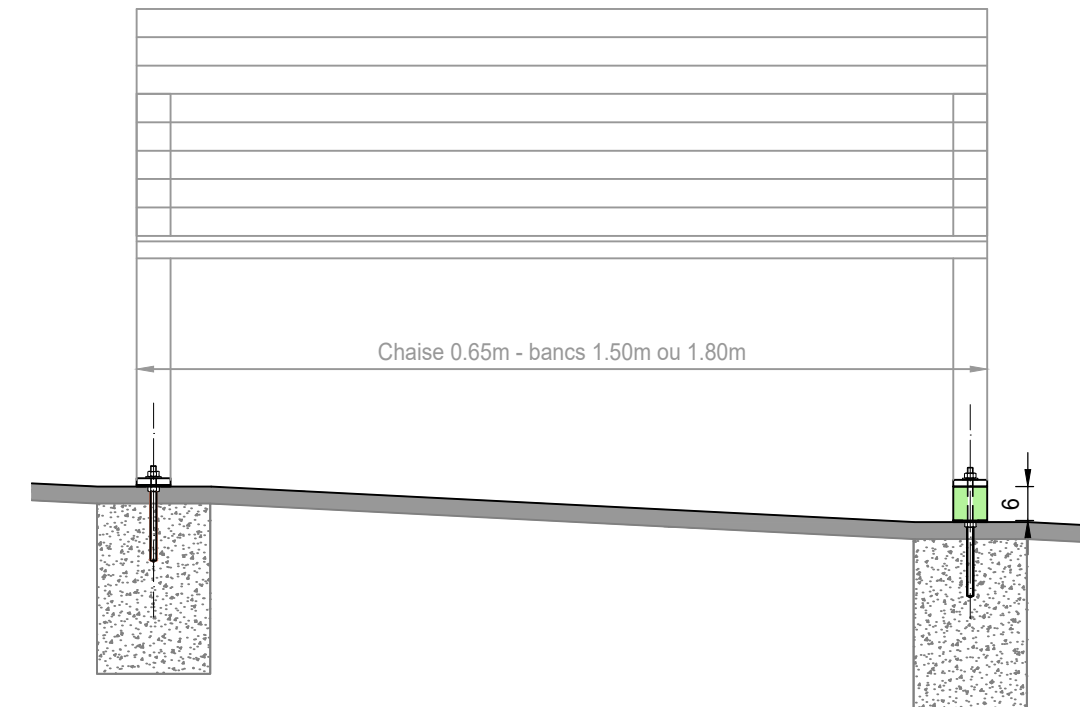
Coupe C - C
